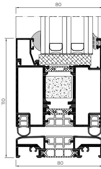
SEZIONE INFERIORE CON SOGLIA
