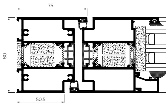
SOLUZIONE CON VETRO
