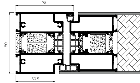
SOLUZIONE CON PANNELLO
